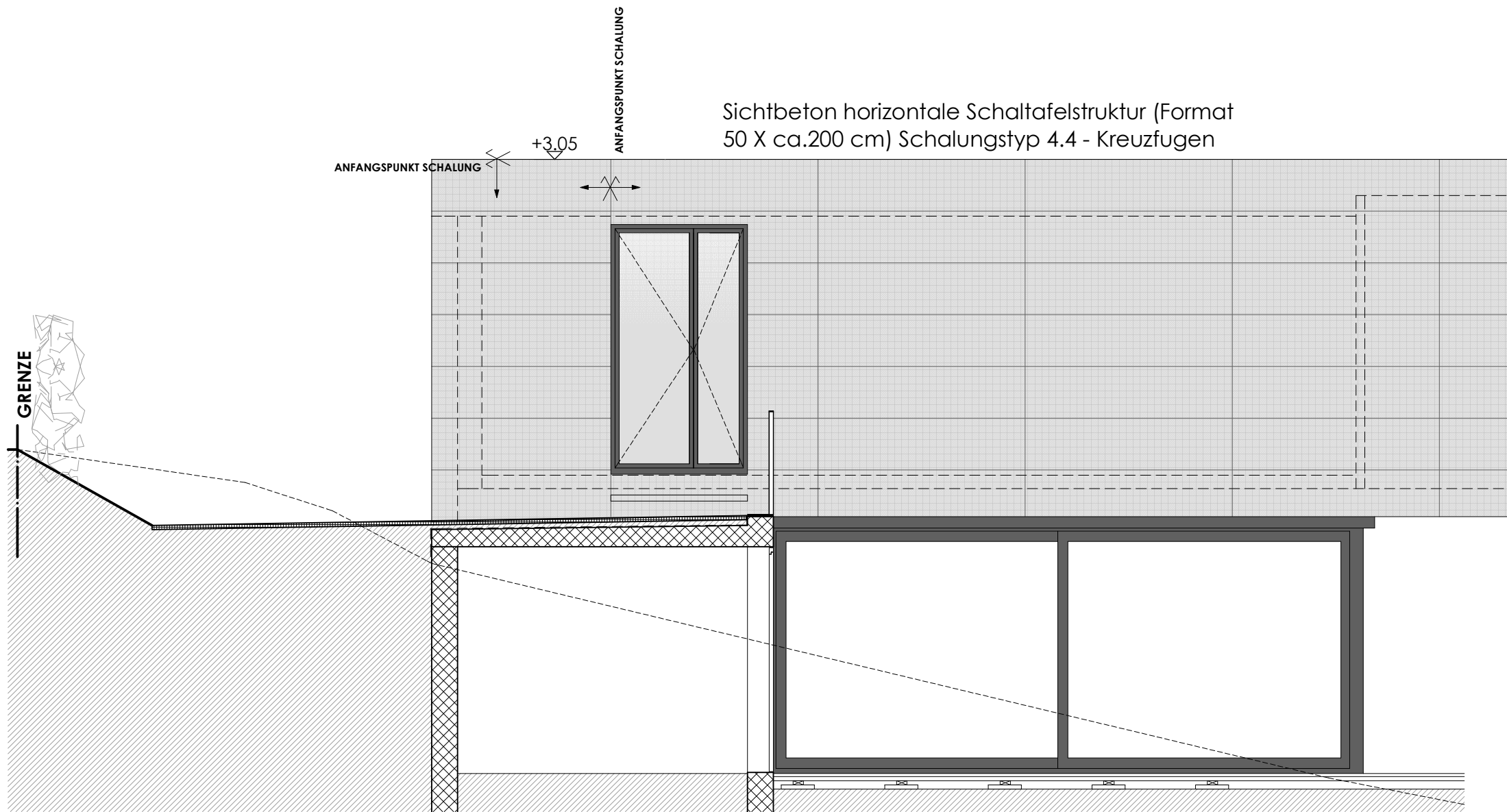
WANDE UMGEBUNG Sichtbeton horizontale Schaltafelstruktur (Format 50 X ca.200 cm) Schalungstyp 4.4 - Kreuzfugen
