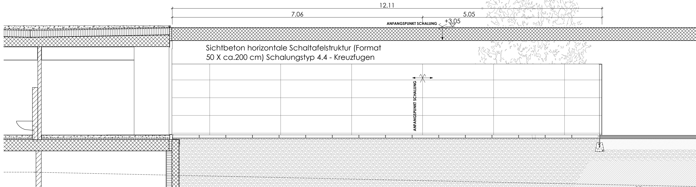
Sichtbeton horizontale Schaltafelstruktur (Format 50 X ca.200 cm) Schalungstyp 4.4 - Kreuzfugen
