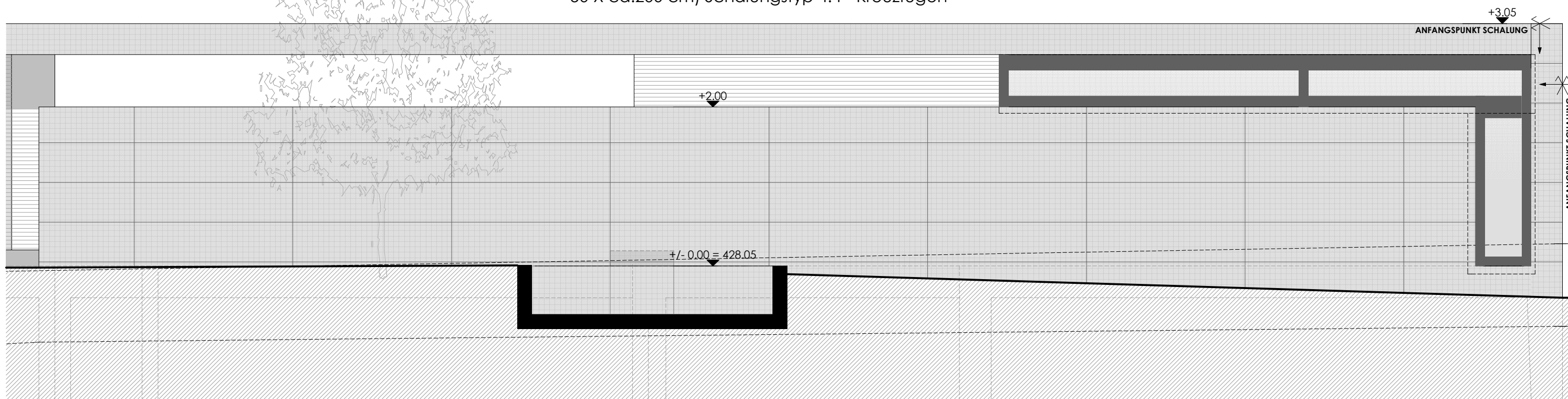
Sichtbeton horizontale Schaltafelstruktur (Format 50 X ca.200 cm) Schalungstyp 4.4 - Kreuzfugen
